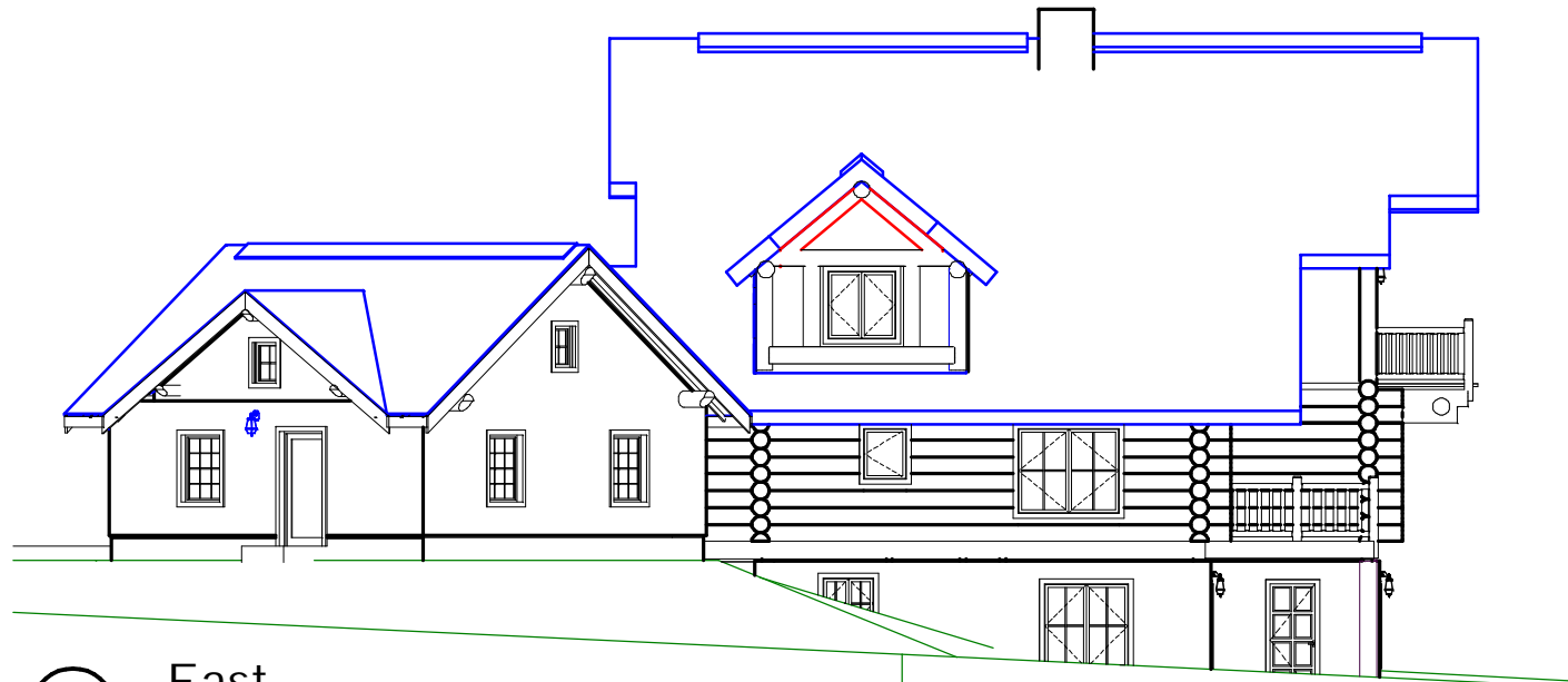
1 East A3 Scale 1/8" = 1' - 0"
